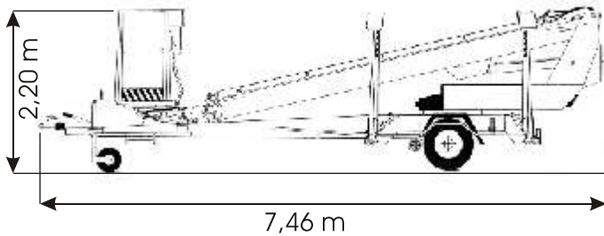
Transportbreite: 1,78 m
